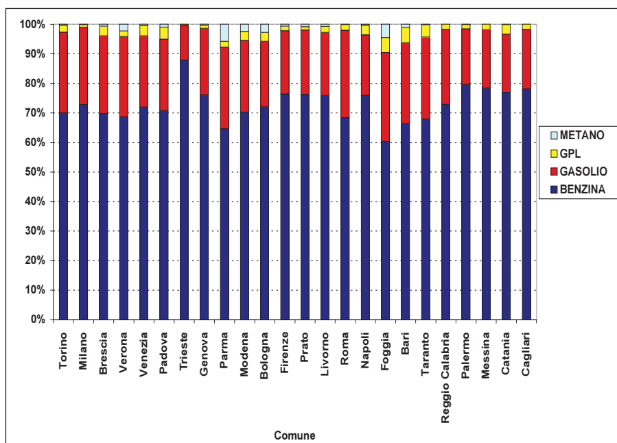
Figura 12: Comuni. Distribuzione percentuale del parco veicolare autoveature per alimentazione. Anno 2004.
