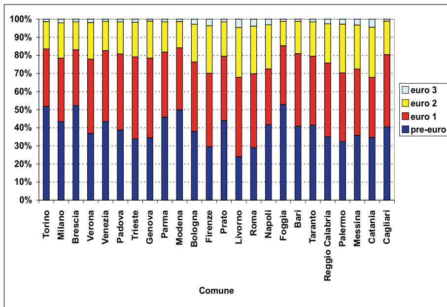
Figura 21: Comuni. Distribuzione percentuale del parco veicolare motocicli per standard emissivo. Anno 2005.
